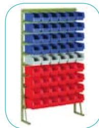
LKV14E 1715 X 1000 mm 54 bacs LKPLK3A
