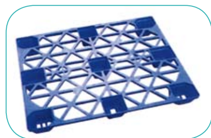
PP100 1200 X 1000 X 145 mm 2500 kg / 1000 kg Encastrable / 9 pieds Parfait pour "one-way delivery"
