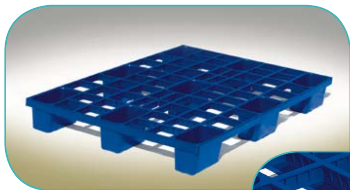
PP80 1200 X 800 X 145 mm 2000 kg / 800 kg Encastrable / 9 pieds
