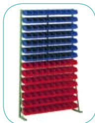
LKN14 1000 X 1725 mm 126 bacs LKM4
