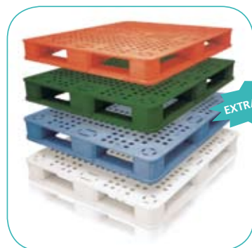
EP1210 - N01 - avec ou sans bord d'empilage 1200 X 1000 X 165 mm 10.000 kg / 2000 kg / 1250 kg
