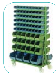
LKNW12FV-versterkt 1000 X 1640 mm 108+36+8 bacs en acier. Charge totale : 650 kg
