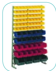
LKV14G 1715 X 1000 mm 27 bacs LKPLK4, 24 LKPLK3, 8 LKPLK2 et 3 LKPLK1
