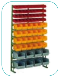
LKN14F 1000 X 1725 mm 36 bacs LKM4, 24 LKM3 et 8 LKM2
