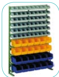
LKN12H 1000 X 1513 mm 54 bacs LKM4, 12 LKM3 et 12 LKM3A
