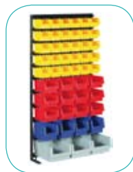
LKV15L 1950 X 1000 mm 30 bacs LKPLK3, 12 LKPLK2, 4 LKPLK2A et 3 LKPLK1
