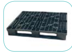
IB100IB 1200 X 1000 X 160 mm (168 mm avec bord) 5000 kg / 1600 kg / 1000 kg
