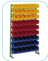
LKN14E 1000 X 1725 mm 45 bacs LKM4 et 36 LKM3
