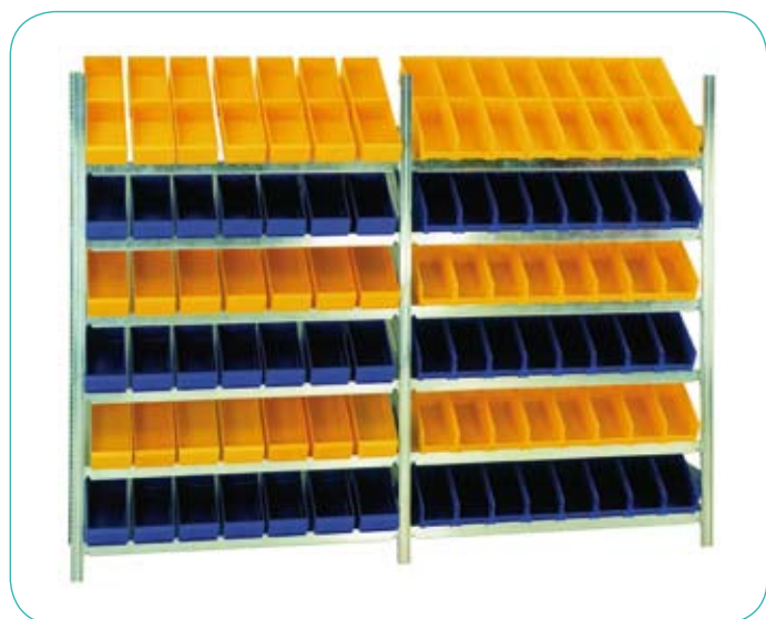
2 exemples avec les mêmes mesures standard. Largeur 1300 mm (X 2), profondeur 1500 mm en hauteur 2000 mm.
