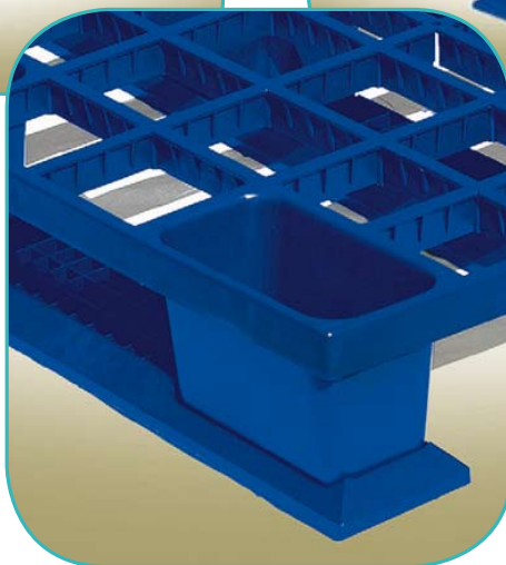
PPS80 1200 X 800 X 145 mm 2500 kg / 1200 kg Niet nestbaar / 3 sleden
