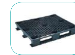
IB100AB 1200 X 1000 X 165 mm (173 mm met rand) 4000 kg / 1200 kg
