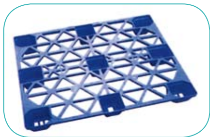
PP100 1200 X 1000 X 145 mm 2500 kg / 1000 kg Nestbaar / 9 voeten Perfect voor "one-way delivery"
