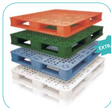
EP1210 - N01 - met of zonder stapelrand 1200 X 1000 X 165 mm 10.000 kg / 2000 kg / 1250 kg
