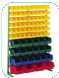
LKN12G 1000 X 1513 mm 54 bakjes LKM4, 12 LKM3, 6 LKM3A en 4 LKM2
