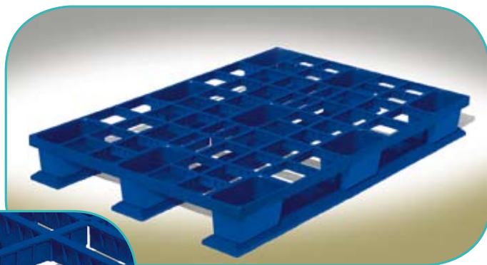
PPS80 1200 X 800 X 145 mm 2500 kg / 1200 kg Niet nestbaar / 3 sleden
