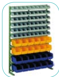
LKN12H 1000 X 1513 mm 54 bakjes LKM4, 12 LKM3 en 12 LKM3A
