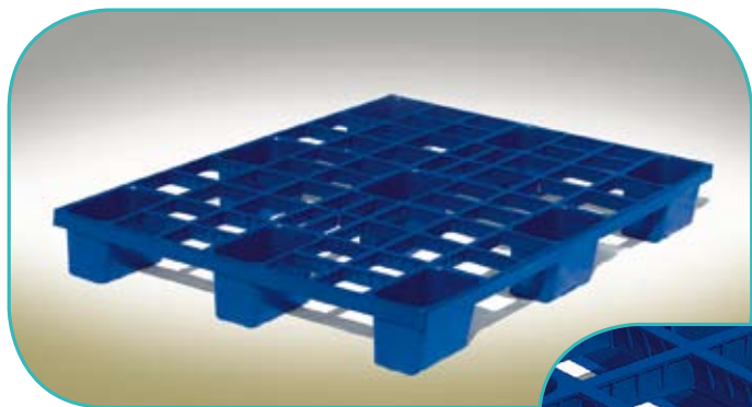
PP80 1200 X 800 X 145 mm 2000 kg / 800 kg Nestbaar / 9 voeten
